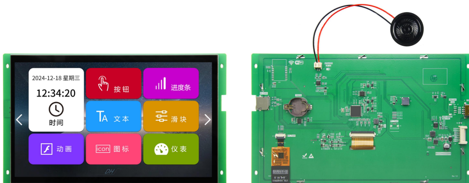
图 1-2 10.1 寸电容触摸参考图
