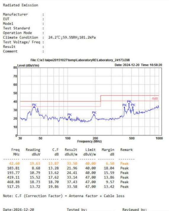
图 4-6 RE 测试垂直方向
