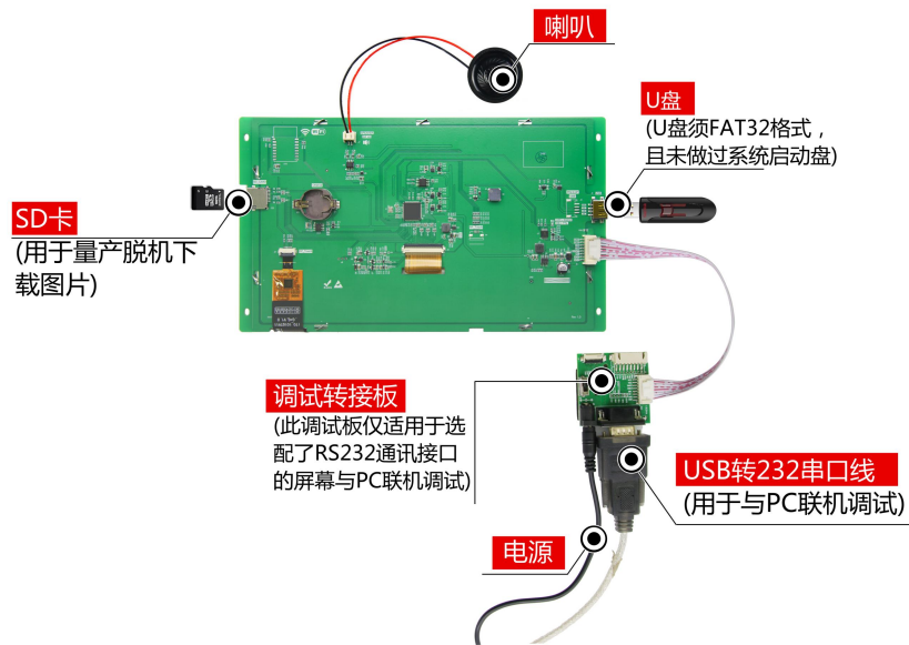
图 1-5 调试工具图
